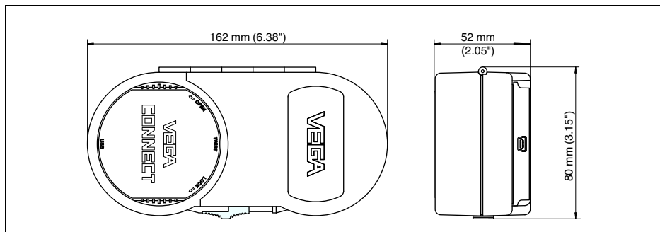
Рис. 12: Размеры VEGACONNECT 4
