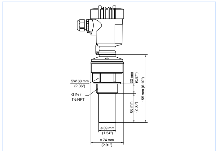
Размеры VEGASON 61
